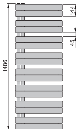
Vorderansicht ROI-150-060
