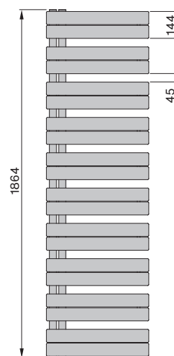
Vorderansicht ROI-180-060
