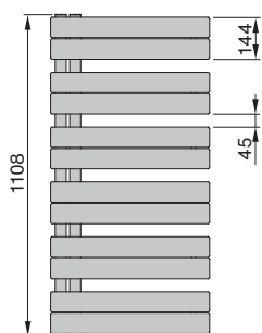
Vorderansicht ROI-120-060
