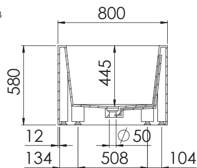
SCHNITT B-B
