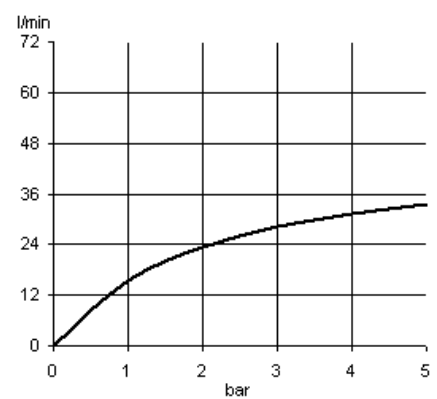
Durchflussdiagramm
