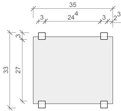
Draufsicht . Top View
