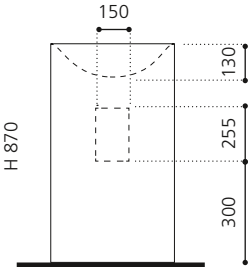
Variante 1: Wandablauf
