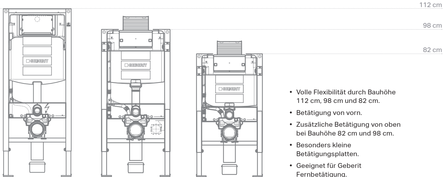
Geberit Unterputz-Spülkasten Omega
