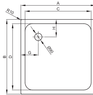
Duschwanne mit Schenkel < 1000 mm
