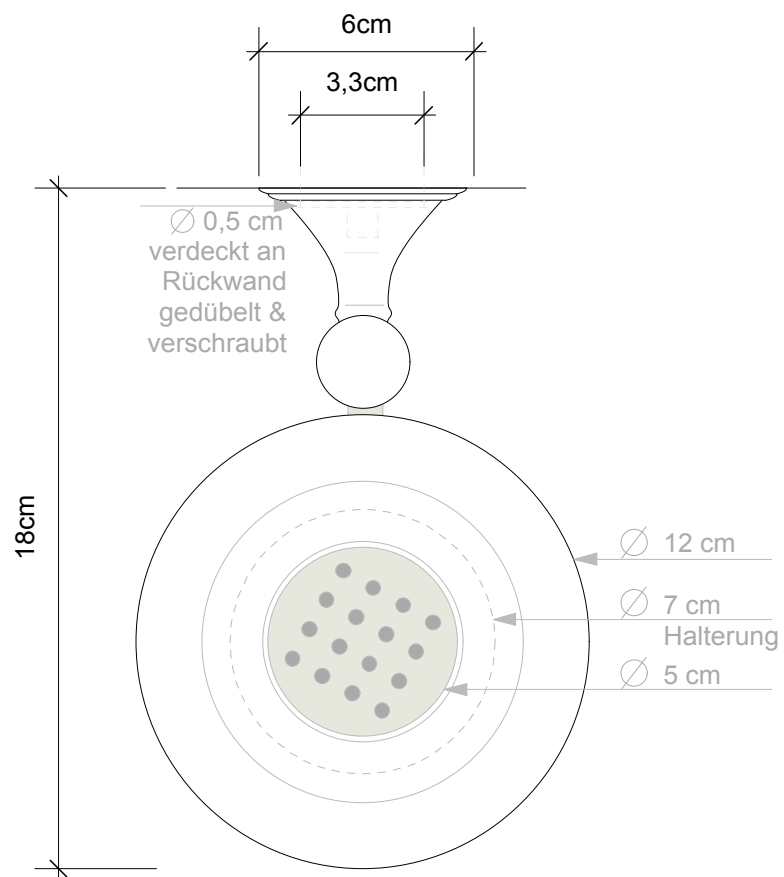
Draufsicht
