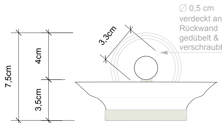
Frontalansicht
