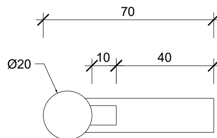
Seitenansicht side view
