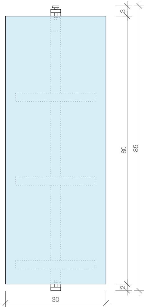
Bohrabstände Drill distances
