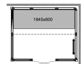
PANACEA 2117 1B Abmessungen: 2125 x 1725 x 2090 mm
