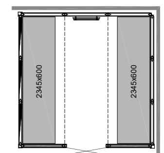
PANACEA 2525 2B Abmessungen: 2525 x 2525 x 2090 mm
