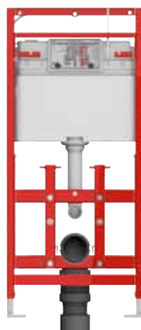
TECElux 200 Best.-Nr. 9600200
