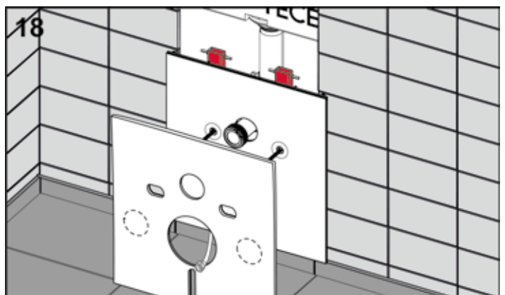
Schallschutzset aufsetzen.
