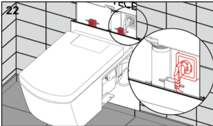
Stromanschluss herstellen: Einstecken des Steckers in die Steckdose.
