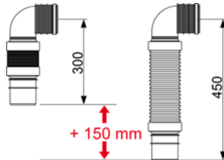
Flexible Längenausdehnung
