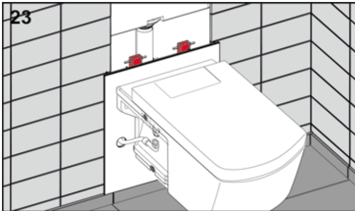
Verbinden des Anschlusspanzerschlauchs mit dem Dusch-WC.
