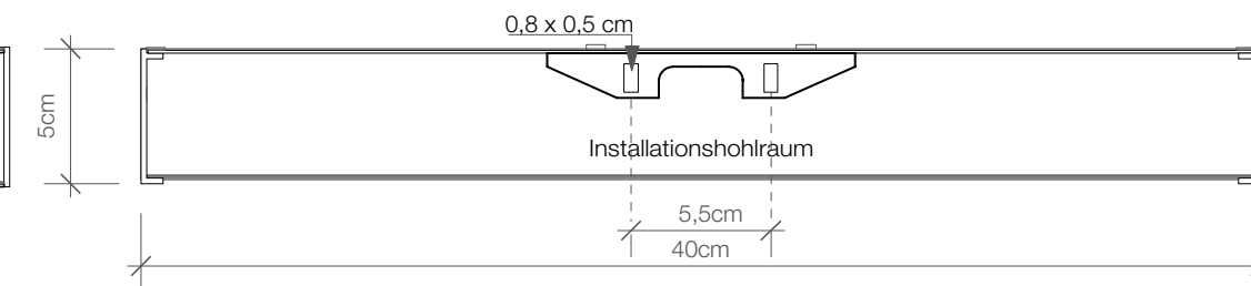
Rückansicht Wandmontage Back view wall fastening
