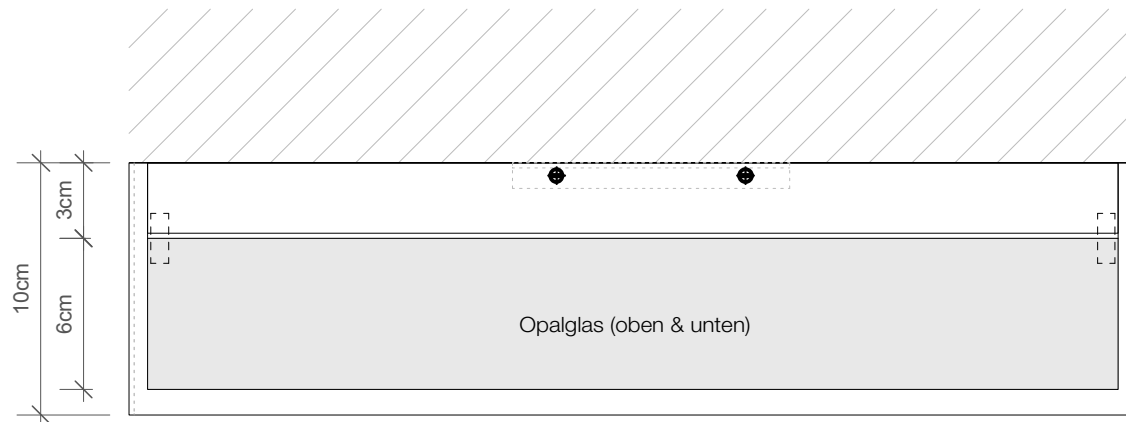
Draufsicht Wandmontage Top view wall fastening
