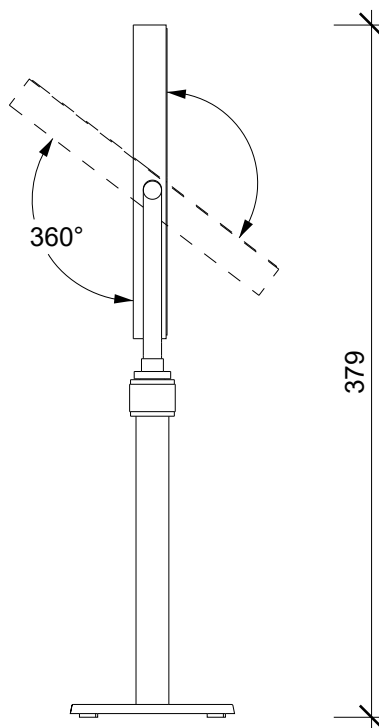
Seitenansicht side view
